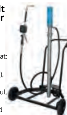
Distribusjonssett for AdBlue® (ORI 55525)
